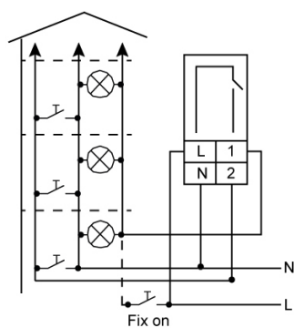
Conexión a 3 hilos 3 wire connection
