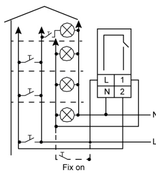
Conexión a 4 hilos 4 wire connection
