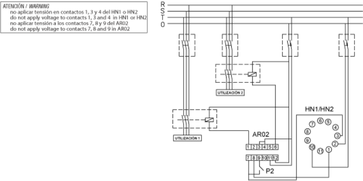
Conexión con interruptores de nivel HN1/HN2 Connection with level control switch HN1/HN2
